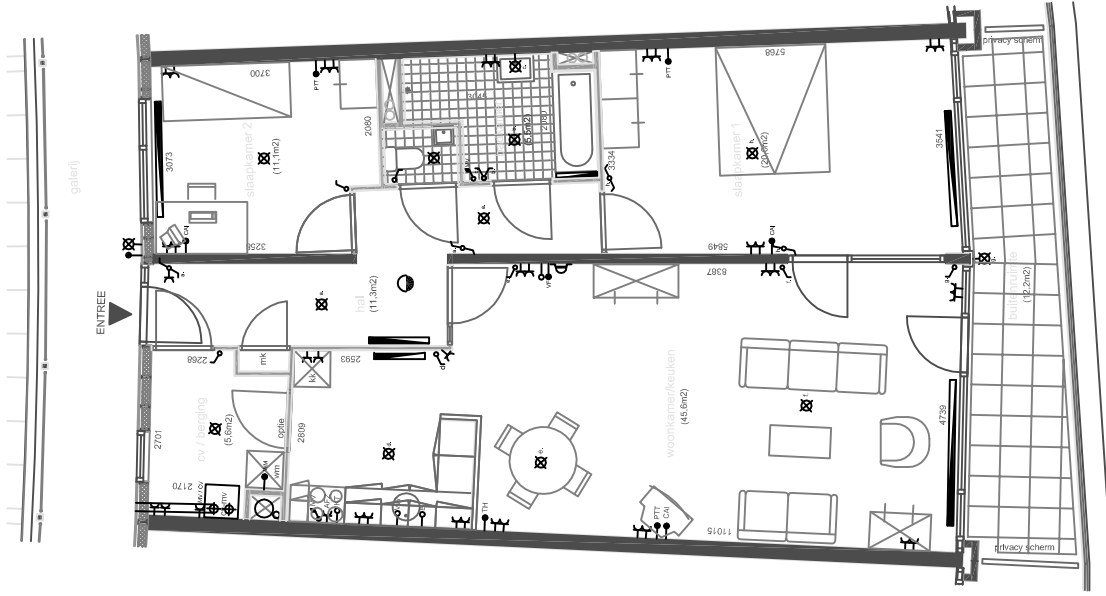
PLATTEGROND TYPE C1 HOLTERWEG SCHAAL 1:50 DATUM: 06-05-2003
