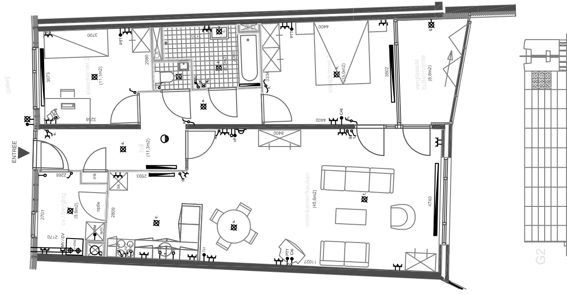
PLATTEGROND TYPE G2 OOSTRIKLAAN SCHAAL 1:50 DATUM: 06-05-2003
